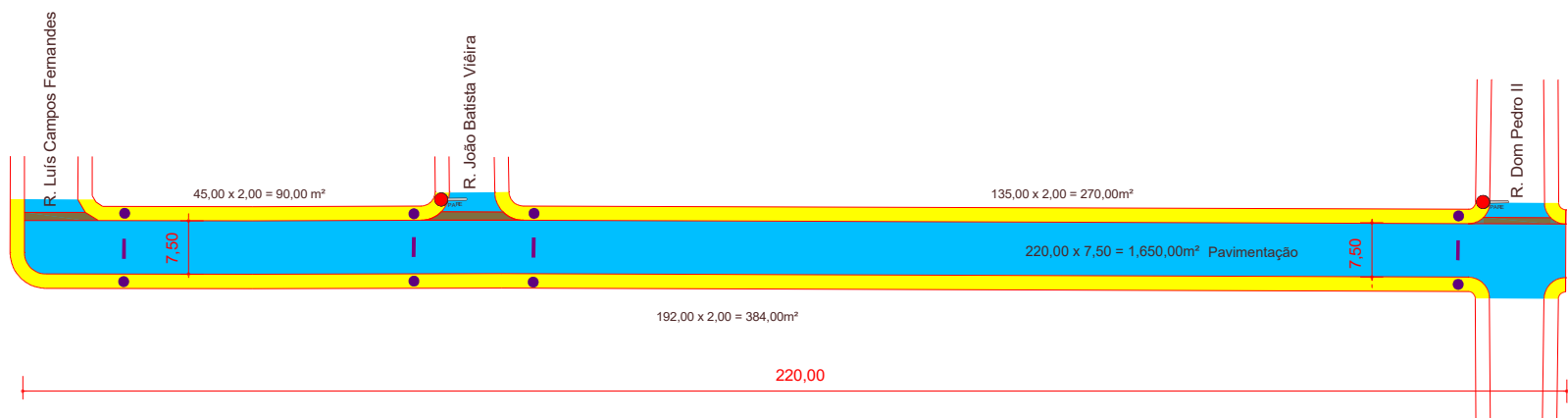
RUA ALEGRE PAVIMENTAÇÃO - Sem escala
