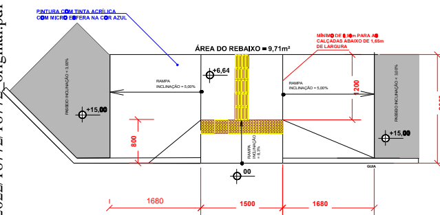
DET. Rampa de Acessibilidade Sem Escala
