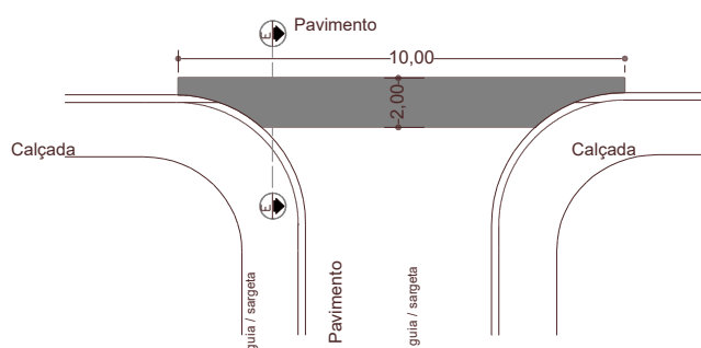
DET. 02 Esquema do "Sarjetão" Sem Escala
