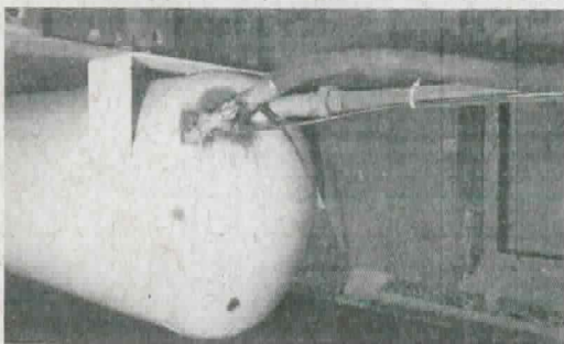
Mangueira (sistema de alimentação de ar do compressor no reservatório) e do lado a válvula de retenção calibra em 130bar.
