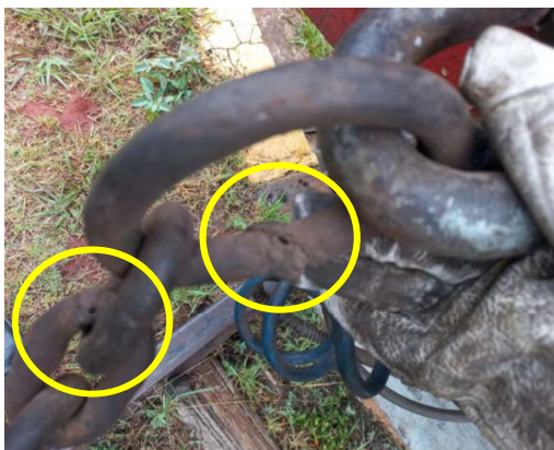
Fig. 5 – Soldas em elos e olhais.
